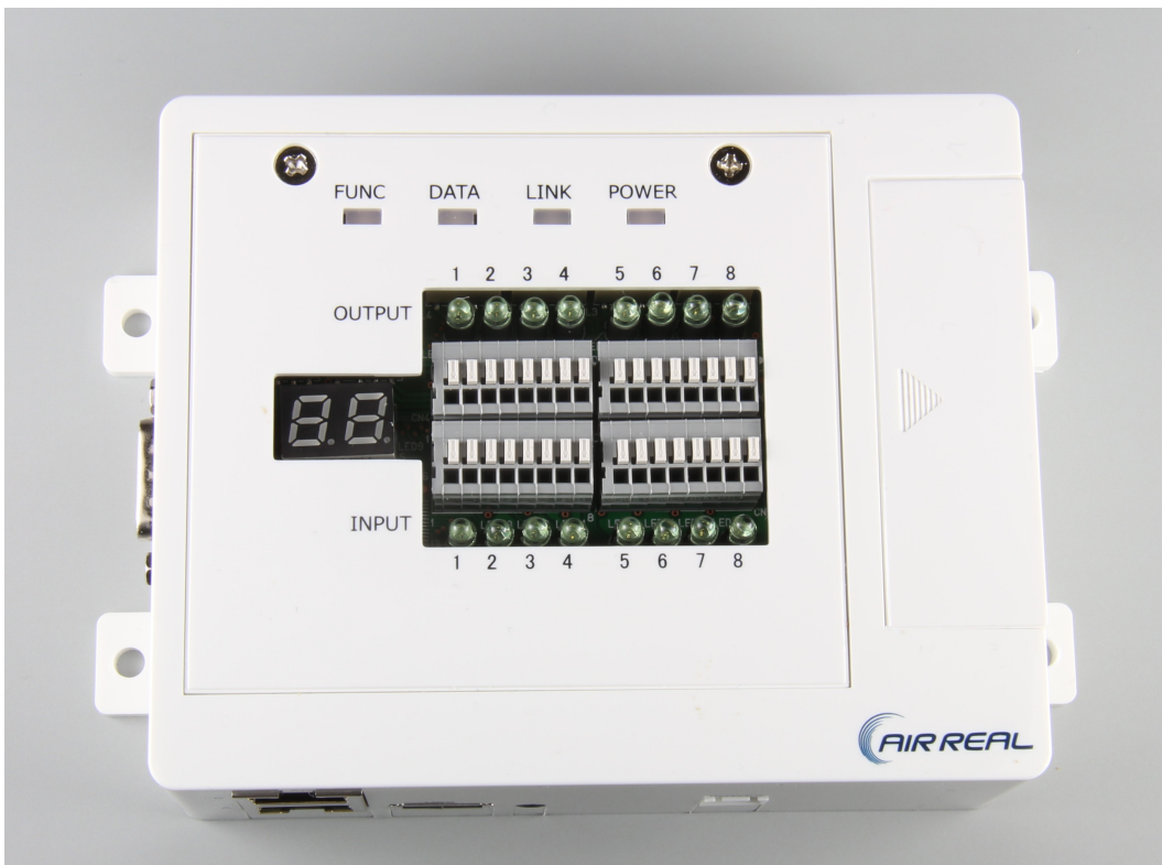
写真3 本体上面
